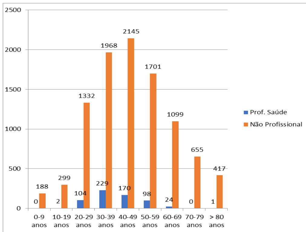
Gráfico 05 – Distribuição dos casos de COVID-19 por faixa etária no município de Nova Iguaçu/RJ – semana epidemiológica 9-52/2020
