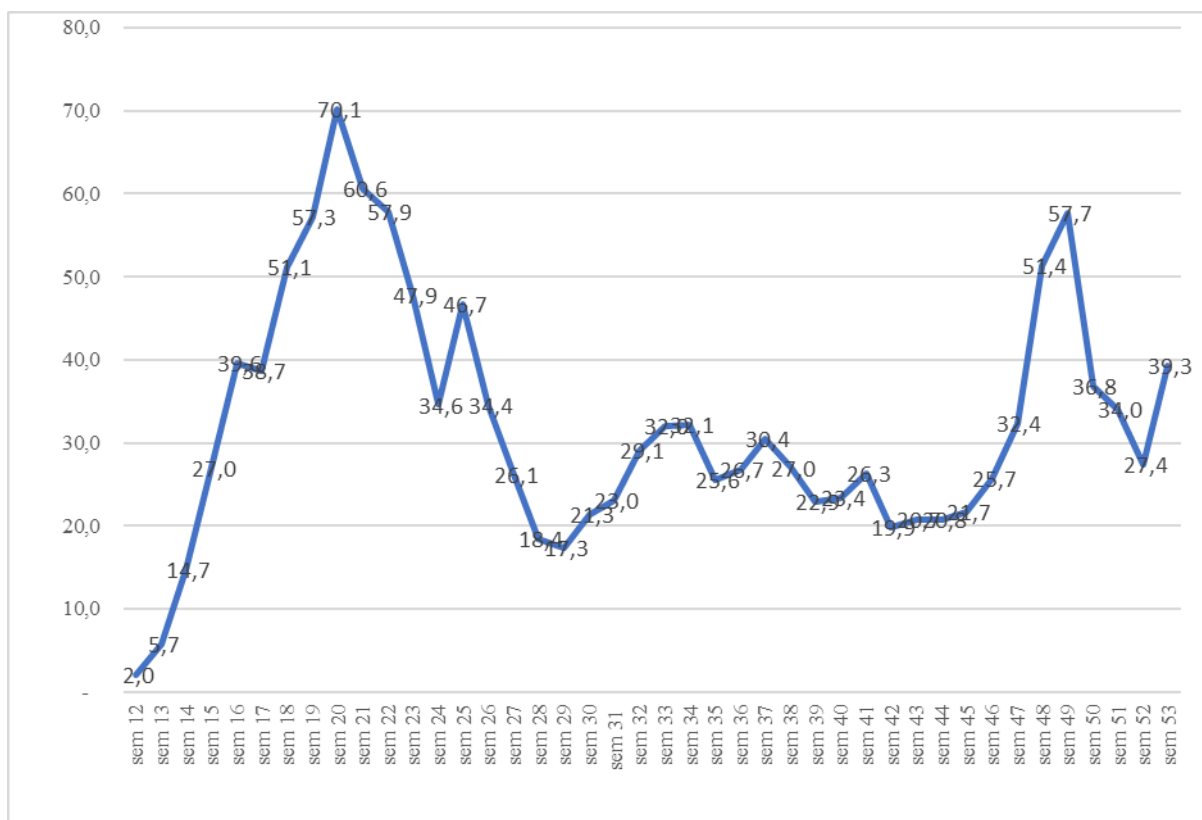
Gráfico 04 – Distribuição da média móvel do número de casos por semana epidemiológica 12-52 no município de Nova Iguaçu/RJ
