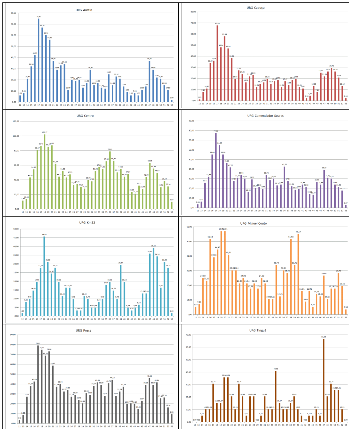
Gráfico 06 - Taxa de incidência de covid19 (100 mil habitantes) segundo URG e semana epidemiológica dos 1º sintomas.
