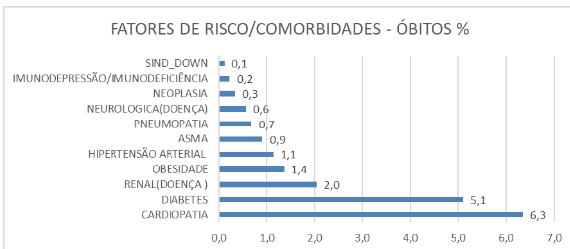
Gráfico 9 - Distribuição de comorbidades entre os óbitos de COVID 19 – Nova Iguaçu/2020
