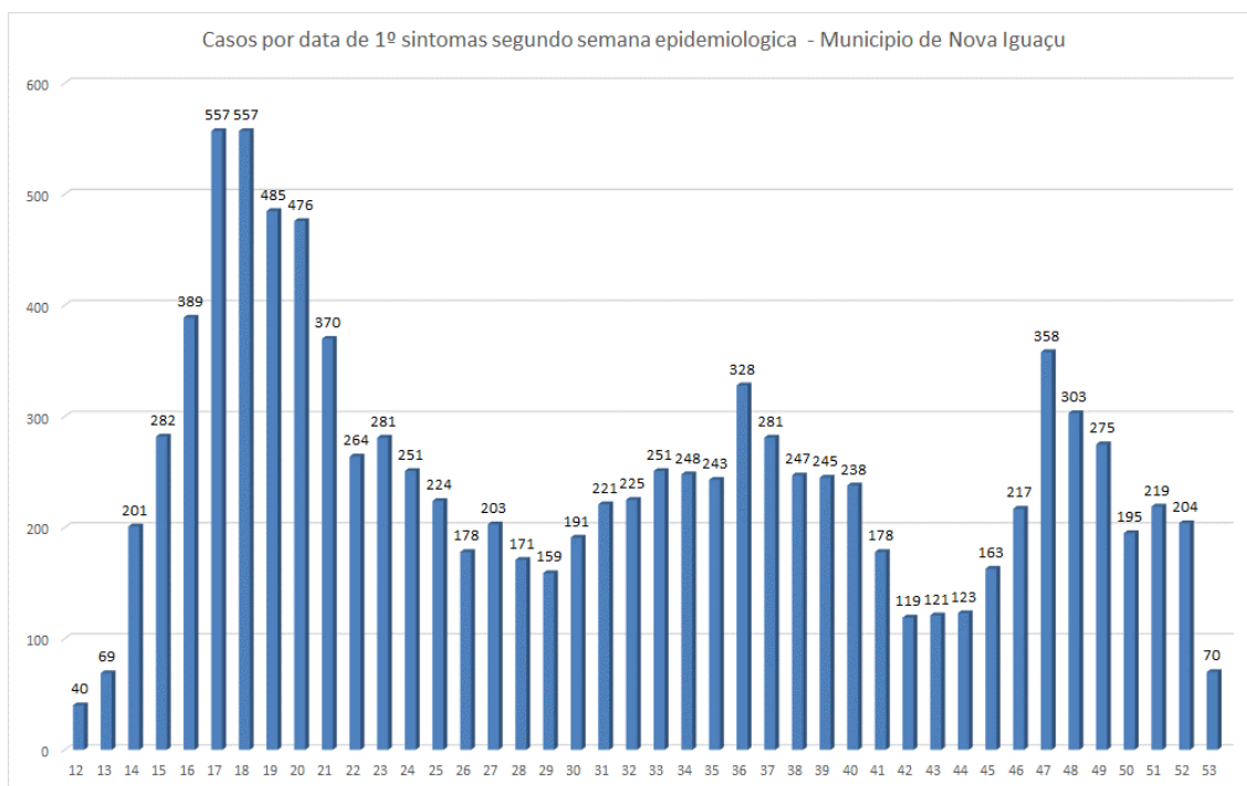
Gráfico 02 - Distribuição de número de casos de COVID-19 de acordo com a data de primeiros sintomas no município de Nova Iguaçu/RJ – Semana Epidemiológica 12-53/2020
