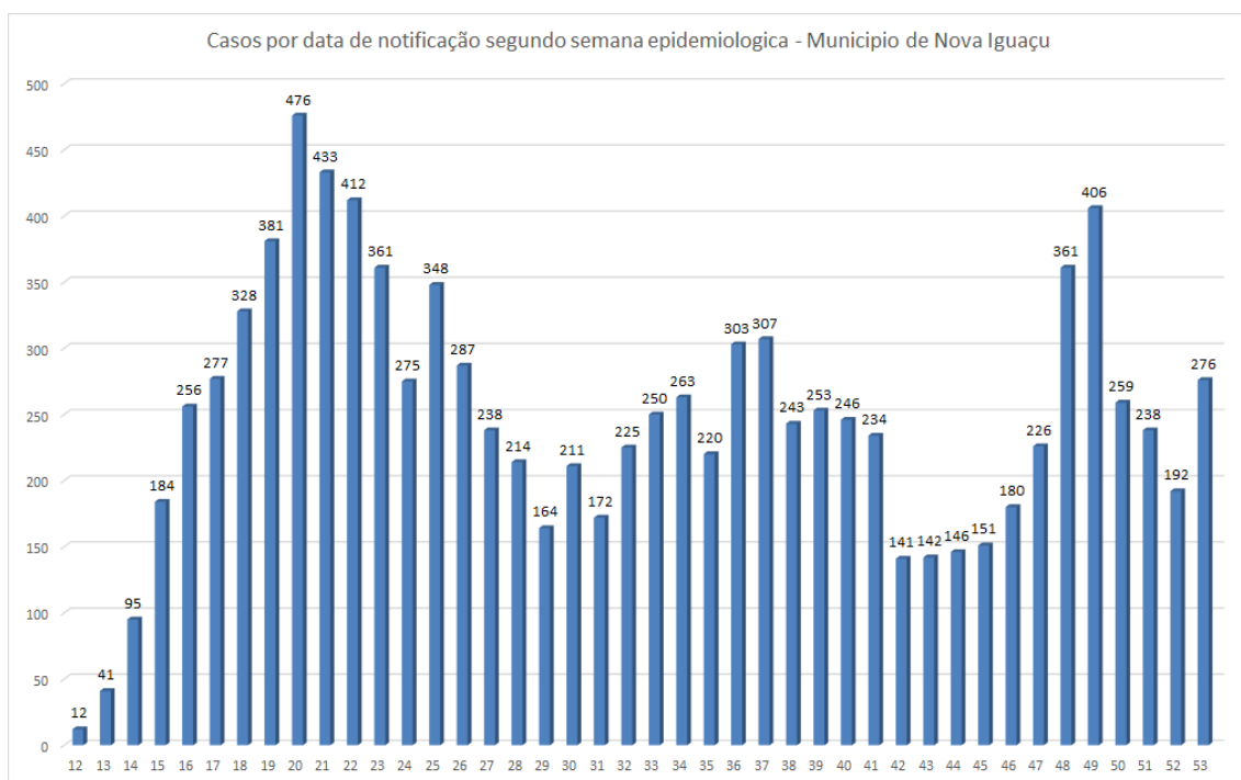
Gráfico 03 - Distribuição de número de casos de COVID-19 de acordo com a data de notificação no município de Nova Iguaçu/RJ – Semana Epidemiológica 12-53/2020
