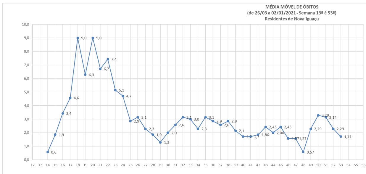
Gráfico 11 – Distribuição da média móvel de óbitos segundo a semana epidemiológica de residentes município Nova Iguaçu (13- 53 semanas)
